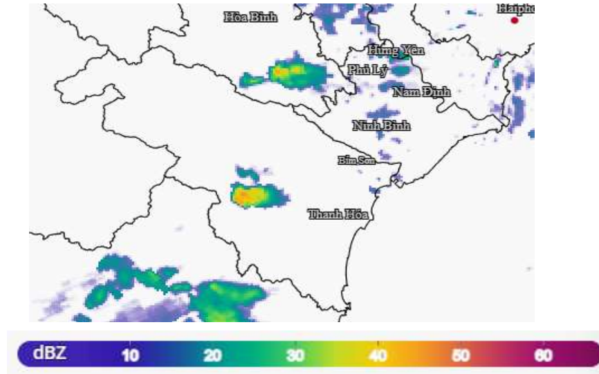
Hình 1: Ảnh radar thời tiết tỉnh Thanh Hóa
