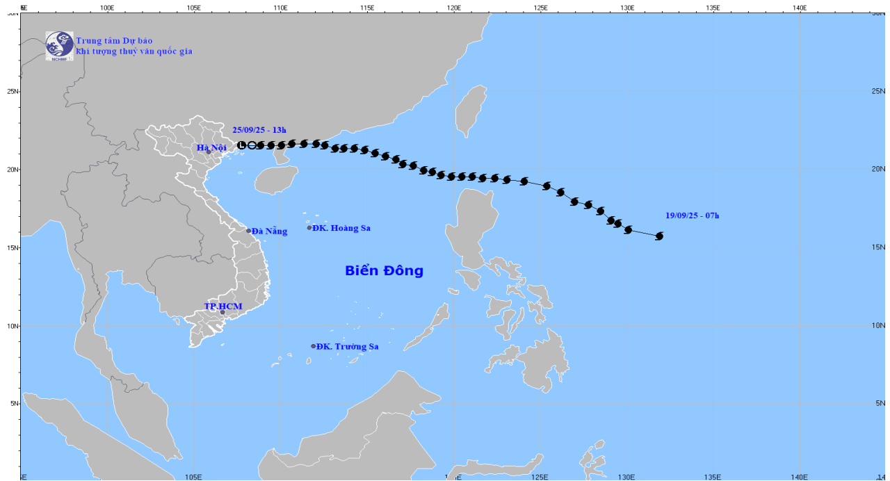
Hình 1. Bản đồ quỹ đạo bão số 9 tính đến 14h00 ngày 25/9/2025 (Nguồn: Trung tâm dự báo KTTV quốc gia)
