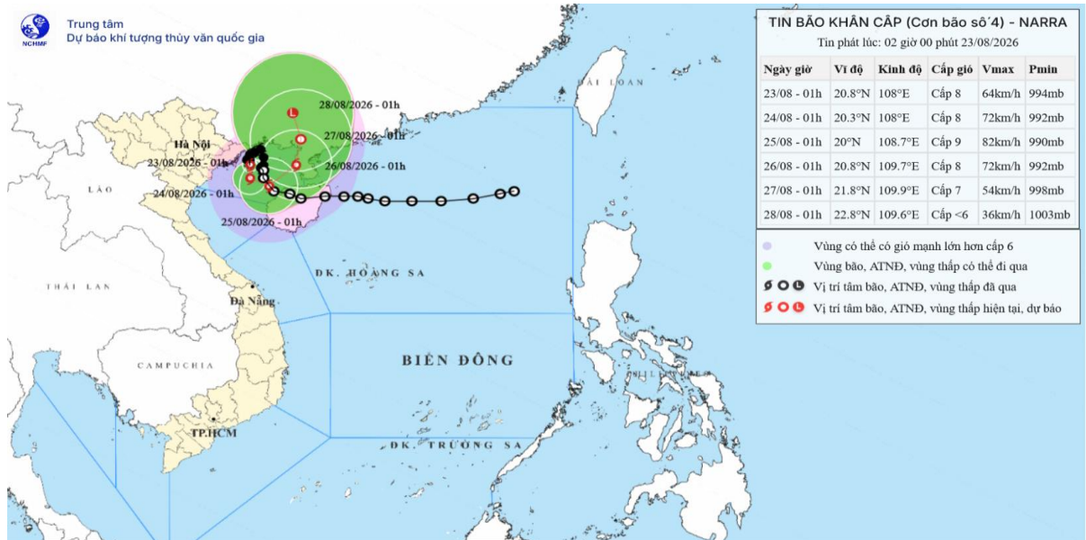
Hình1. Bản đồ dự báo quỹ đạo và cường độ bão số 04 lúc 02h00' ngày 23/8/2026
