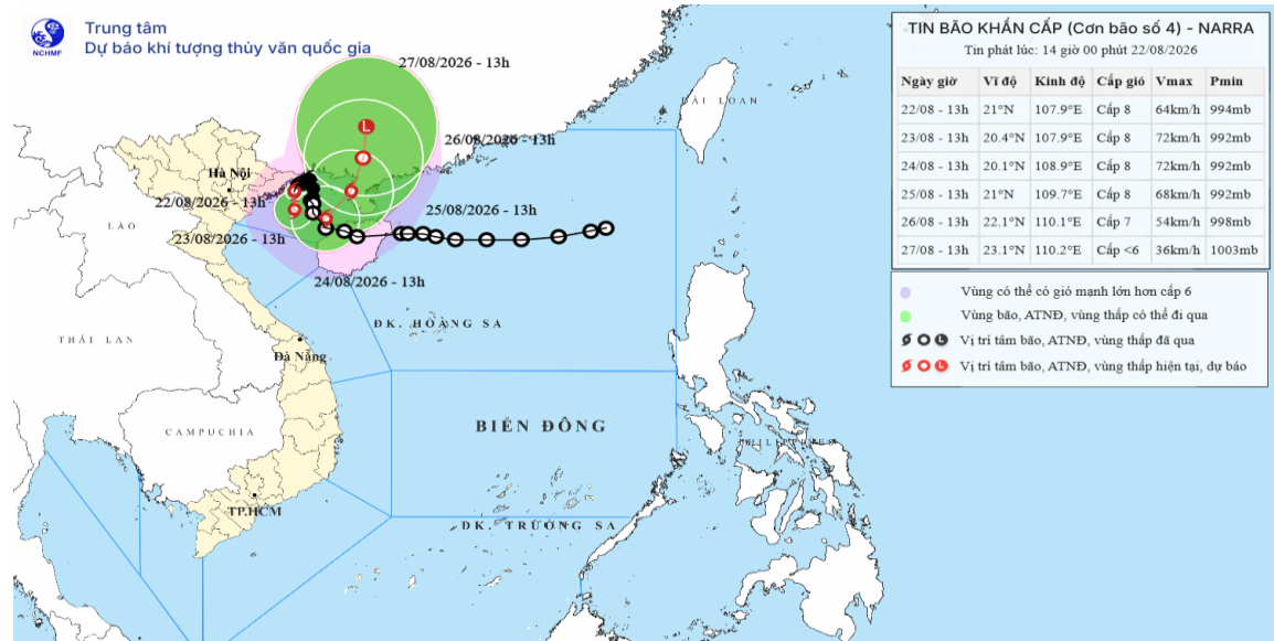
Hình1. Bản đồ dự báo quỹ đạo và cường độ bão số 04 lúc 14h00' ngày 22/8/2026
