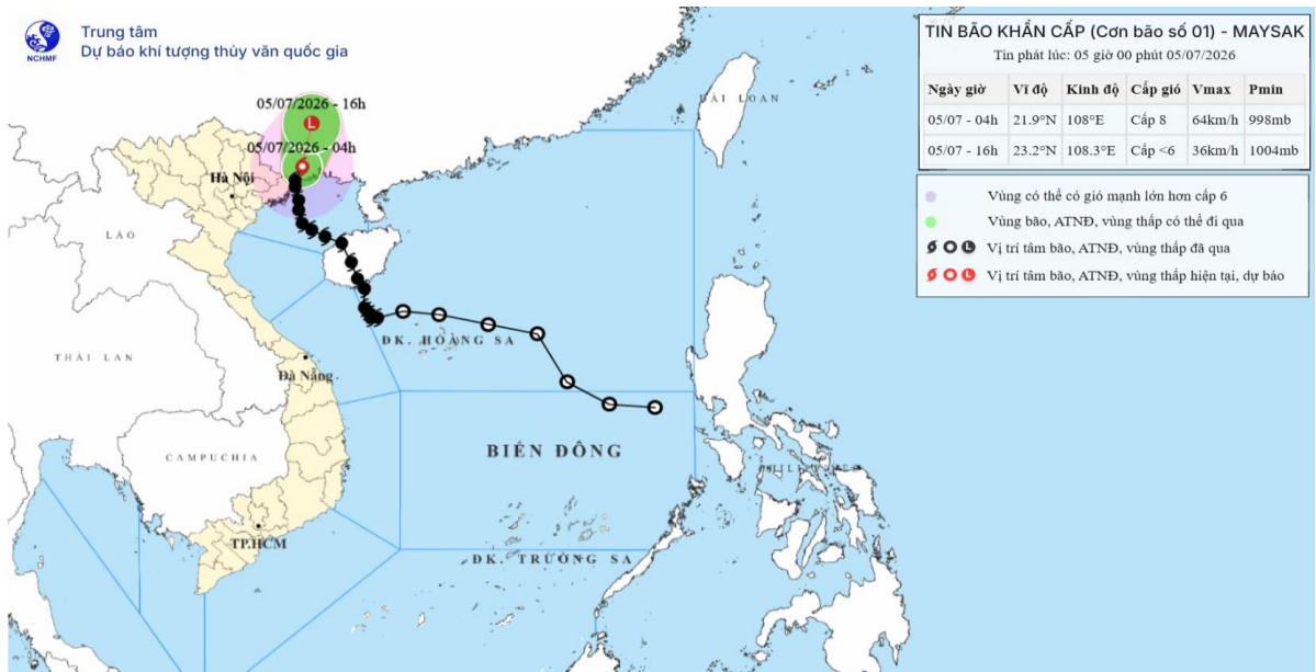
Hình1. Bản đồ dự báo quỹ đạo và cường độ bão số 01 lúc 05h00' ngày 05/7/2026 (Nguồn: Trung tâm dự báo KTTV quốc gia)
