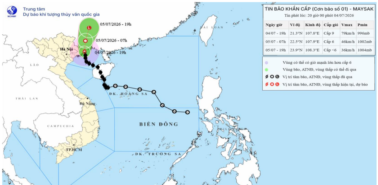
Hình1. Bản đồ dự báo quỹ đạo và cường độ bão số 01 lúc 20h00' ngày 04/7/2026 (Nguồn: Trung tâm dự báo KTTV quốc gia)
