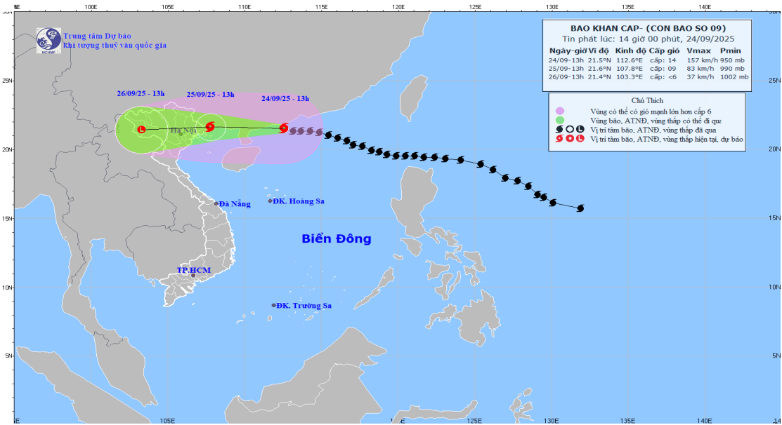
Hình1. Bản đồ dự báo quỹ đạo và cường độ siêu bão số 9 phát lúc 14h00 ngày 24/9/2025 (Nguồn: Trung tâm dự báo KTTV quốc gia)
