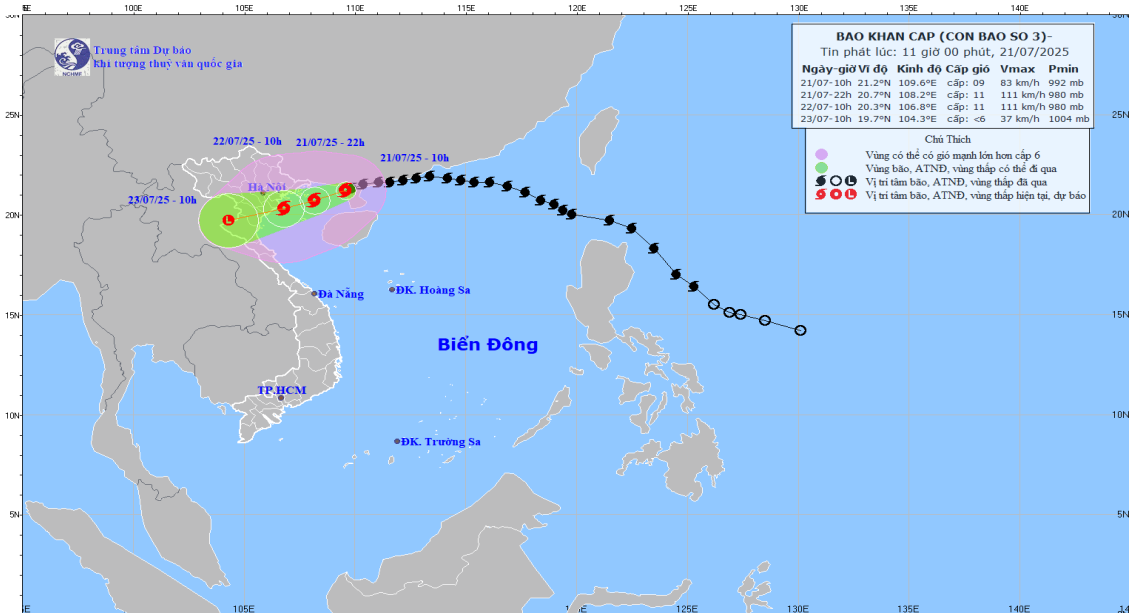
Hình1. Bản đồ dự báo quỹ đạo và cường độ bão số 03 lúc 11h00 ngày 21/7/2025 (Nguồn: Trung tâm dự báo KTTV quốc gia)
