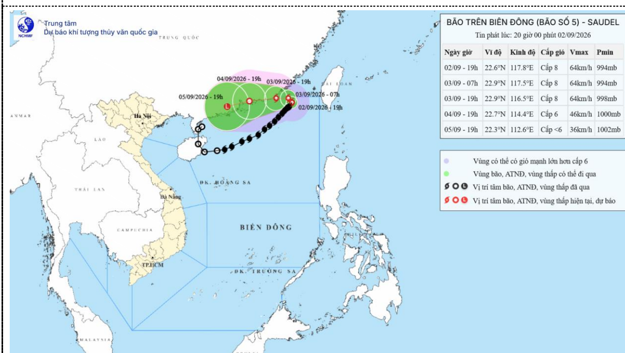
Hình 1. Bản đồ dự báo quỹ đạo và cường độ bão số 05 phát lúc 20h00 ngày 02/9/2026
