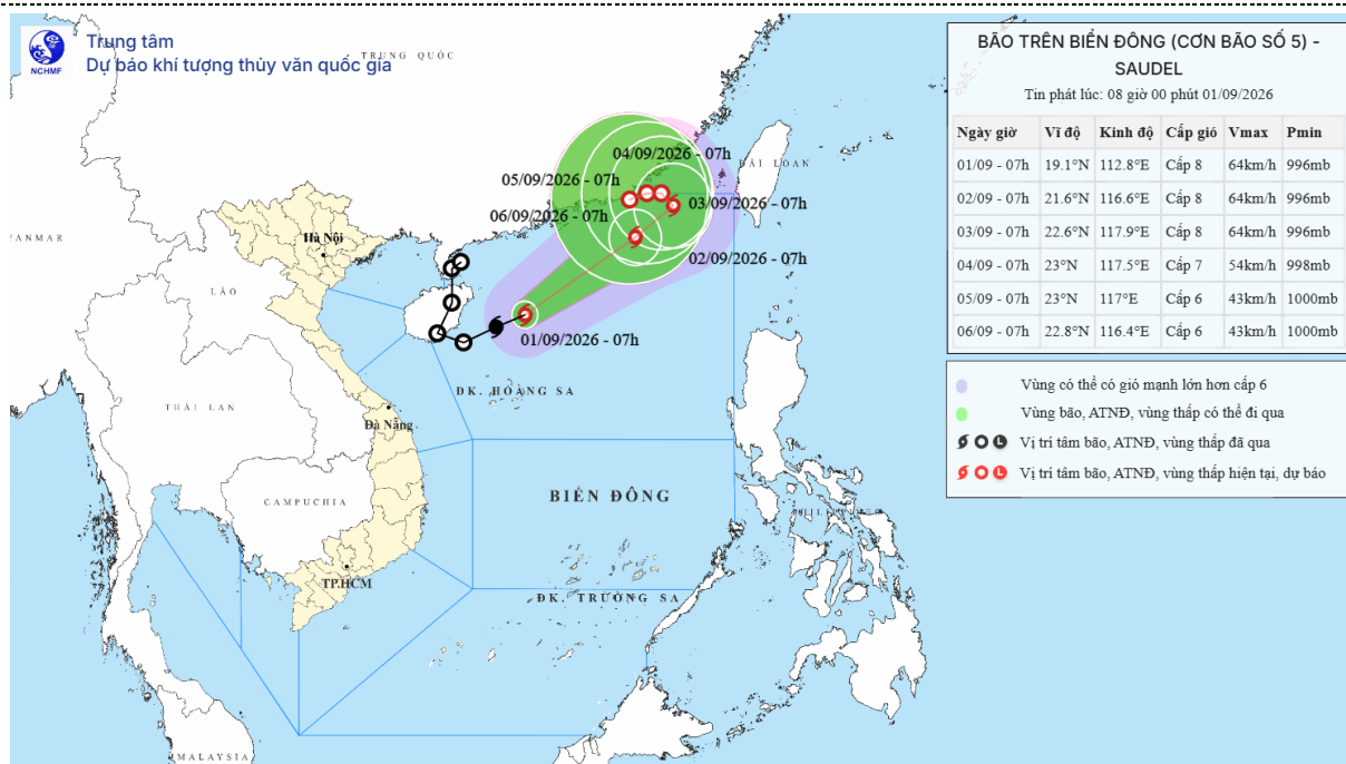
Hình 1. Bản đồ dự báo quỹ đạo và cường độ bão số 05 phát lúc 08h00 ngày 01/9/2026
