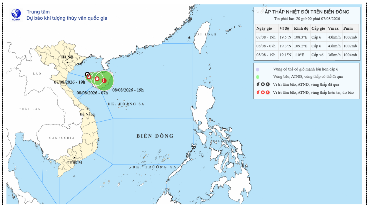
Hình 1. Bản đồ dự báo quỹ đạo và cường độ áp thấp nhiệt đới lúc 20h00 ngày 07/8/2026
