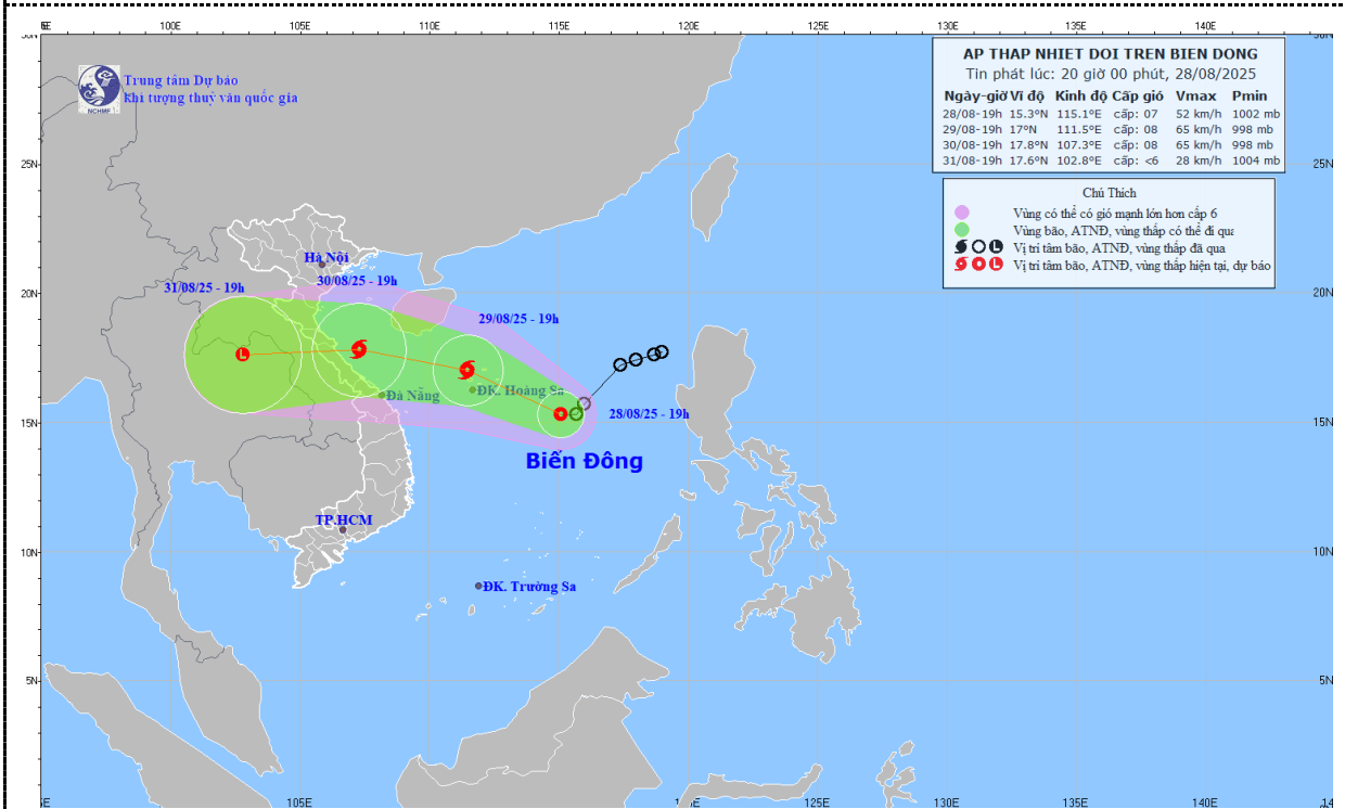
Hình1. Bản đồ dự báo quỹ đạo và cường độ áp thấp nhiệt đới lúc 20h00 ngày 28/8/2025
