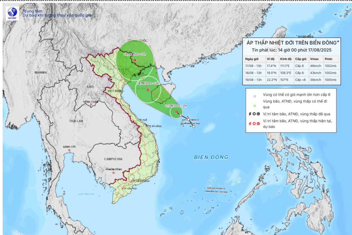
Hình1. Bản đồ dự báo quỹ đạo và cường độ áp thấp nhiệt đới lúc 14h00 ngày 17/8/2025
