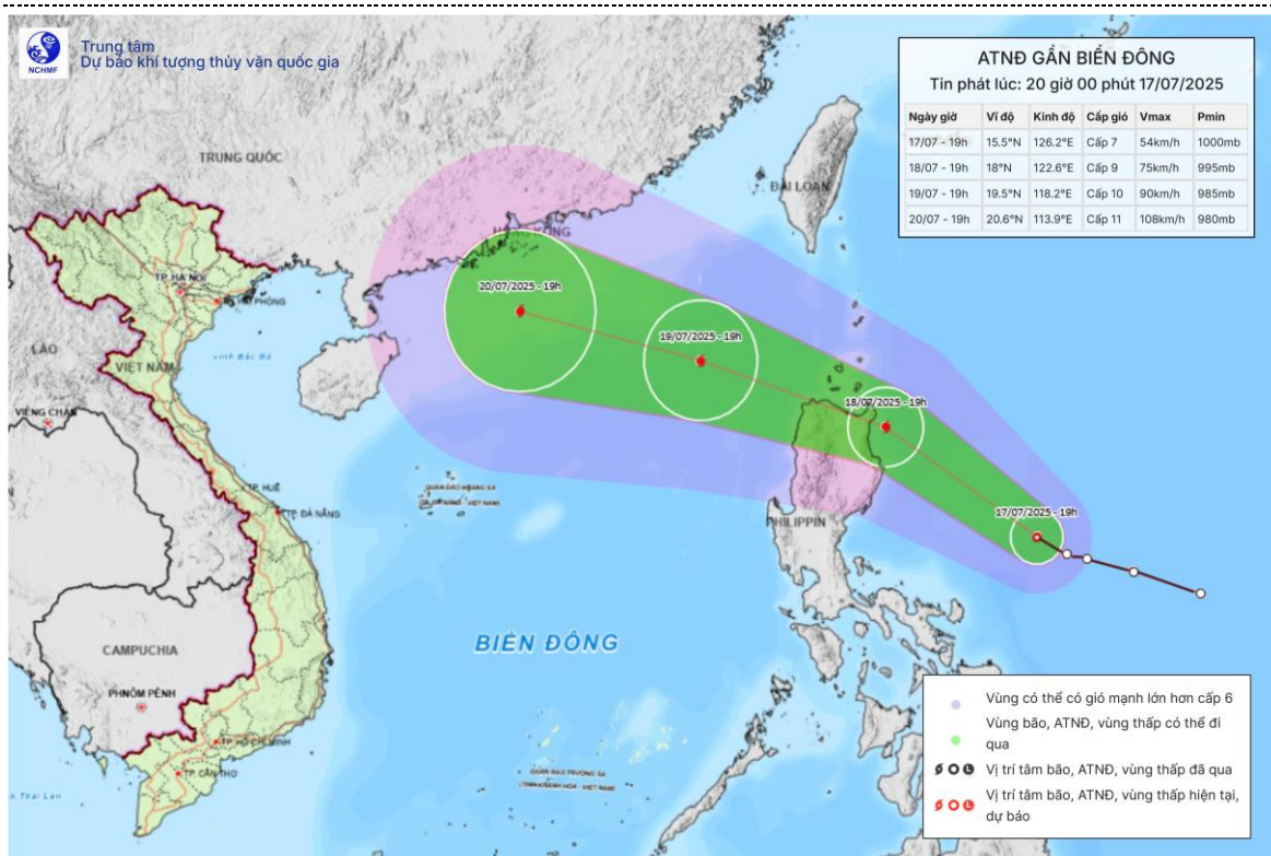
Hình1. Bản đồ dự báo quỹ đạo và cường độ áp thấp nhiệt đới gần Biển Đông phát lúc 20h00 ngày 17/7/2025
