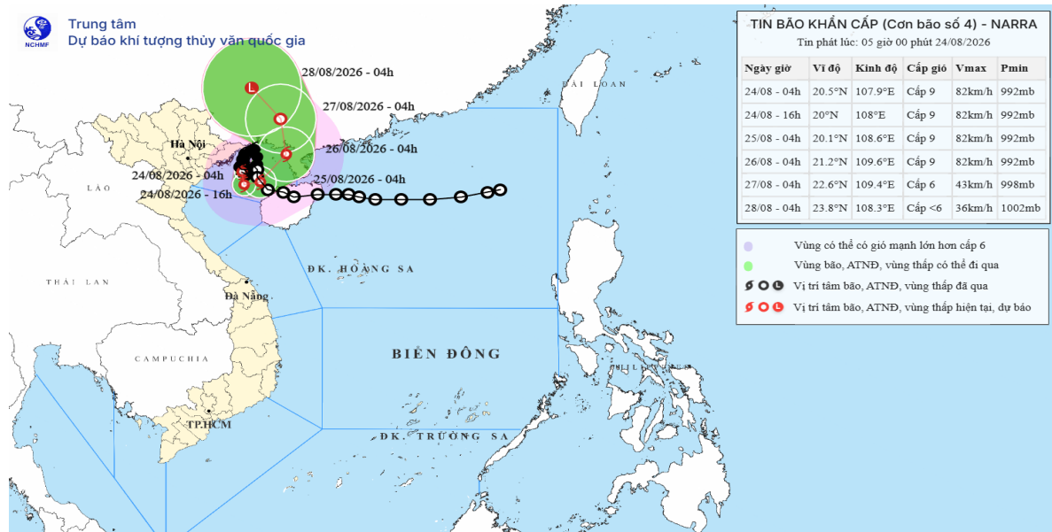
Hình1. Bản đồ dự báo quỹ đạo và cường độ bão số 04 lúc 05h00' ngày 24/8/2026
