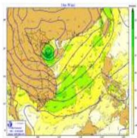
Hình 1: Bản đồ dự báo gió mạnh trong 24 giờ tới
