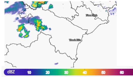
Hình 1: Ảnh radar thời tiết tỉnh Thanh Hóa
