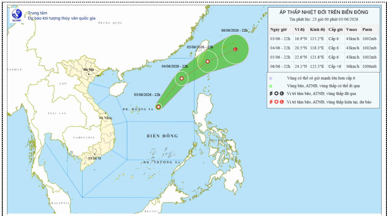
Hình1. Bản đồ dự báo quỹ đạo và cường độ áp thấp nhiệt đới lúc 23h00 ngày 03/6/2026
