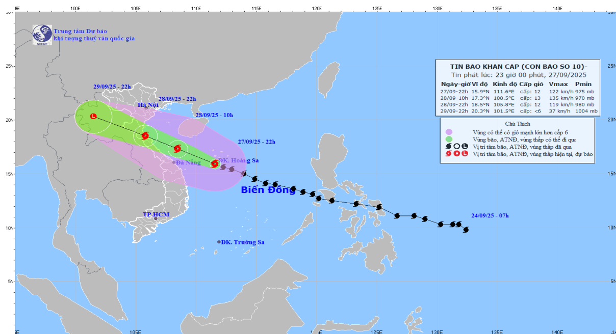
Hình1. Bản đồ dự báo quỹ đạo và cường độ bão số 10 - phát lúc 23h00 ngày 27/9/2025
