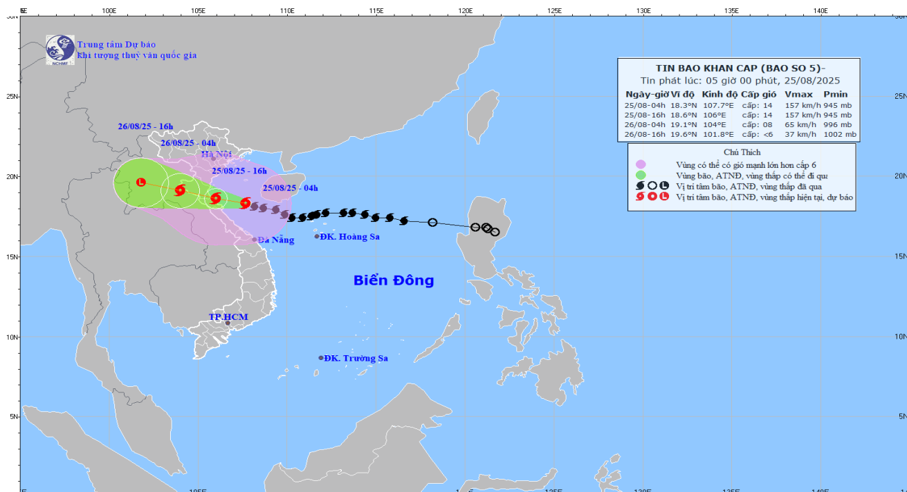
Hình 1. Bản đồ dự báo quỹ đạo và cường độ bão số 05 phát lúc 05h00 ngày 25/8/2025
