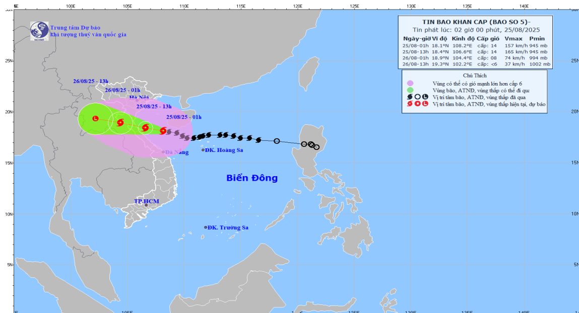
Hình1. Bản đồ dự báo quỹ đạo và cường độ bão số 05 phát lúc 02h00 ngày 25/8/2025
