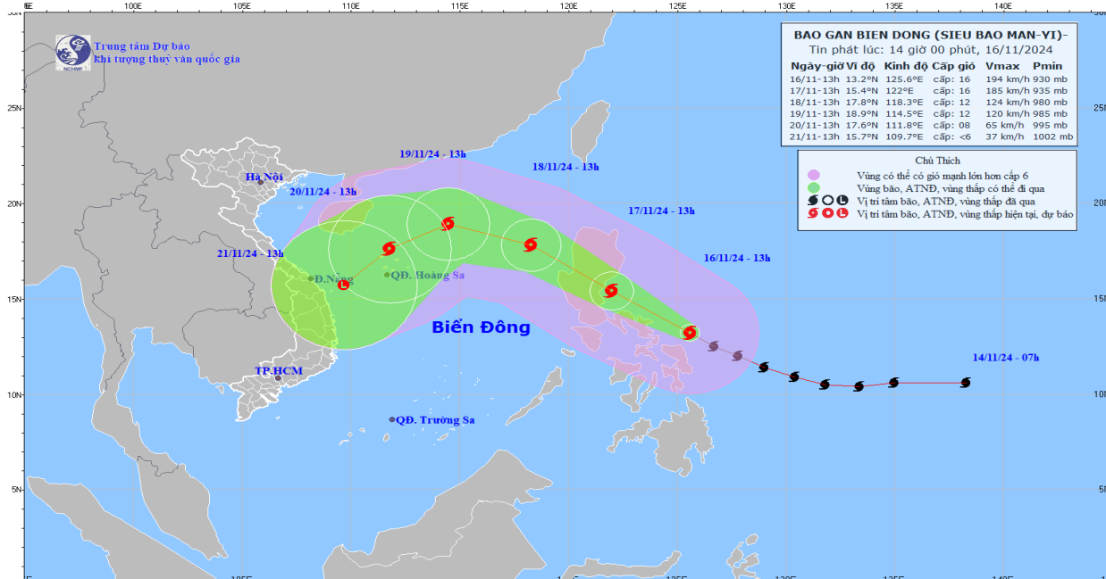
Bản đồ dự báo quỹ đạo và cường độ của siêu bão Man_Yi, phát lúc 14h00, ngày 16/11/2024
