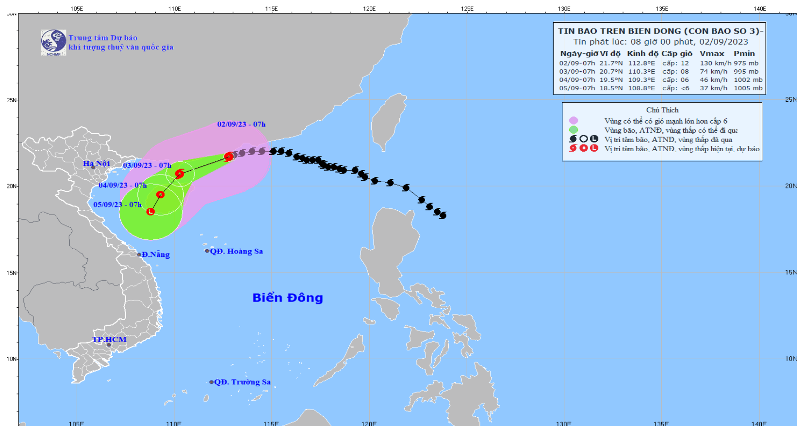
Bản đồ dự báo quỹ đạo và cường độ bão số 3, lúc 08h00 ngày 02/9/2023
