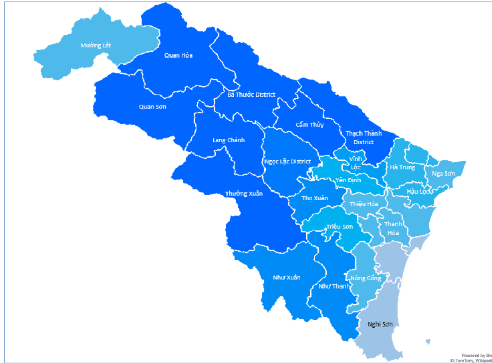
Hình 1: Bản đồ dự báo mưa từ 16h/23/8 đến 16h/24/8/2023
