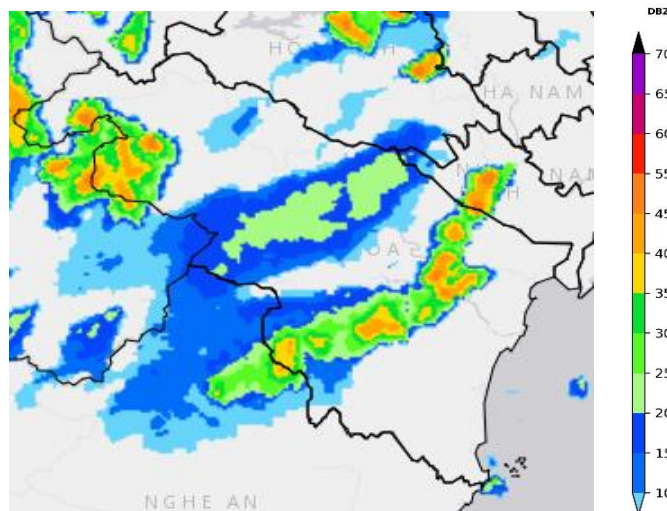
Sản phẩm của Radar lúc 15h30
