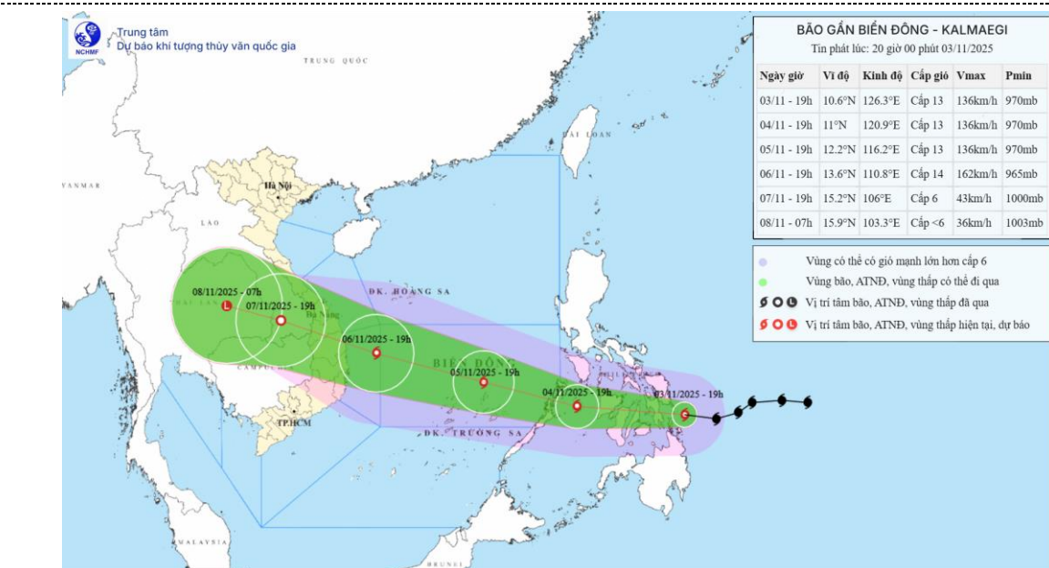
Hình 1. Bản đồ dự báo quỹ đạo và cường độ bão KALMAEGI phát lúc 20h00 ngày 03/11/2025
