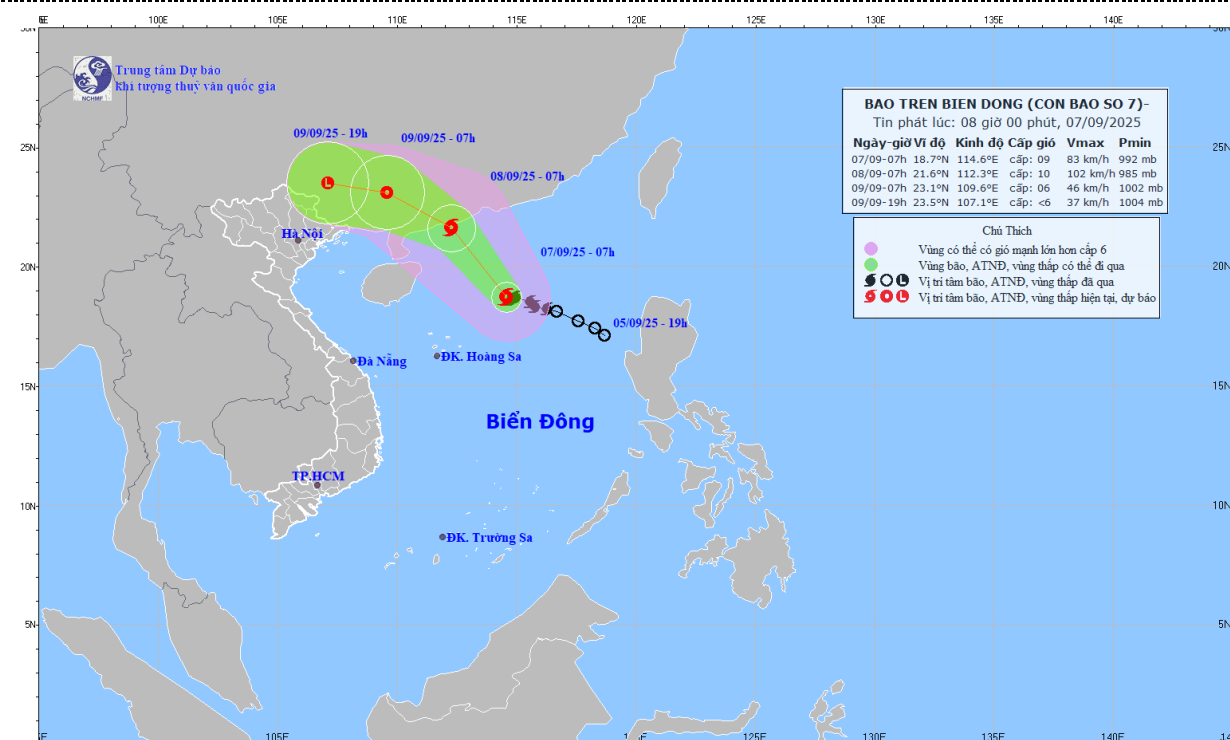
Hình1. Bản đồ dự báo quỹ đạo và cường độ bão lúc 08h00 ngày 07/9/2025
