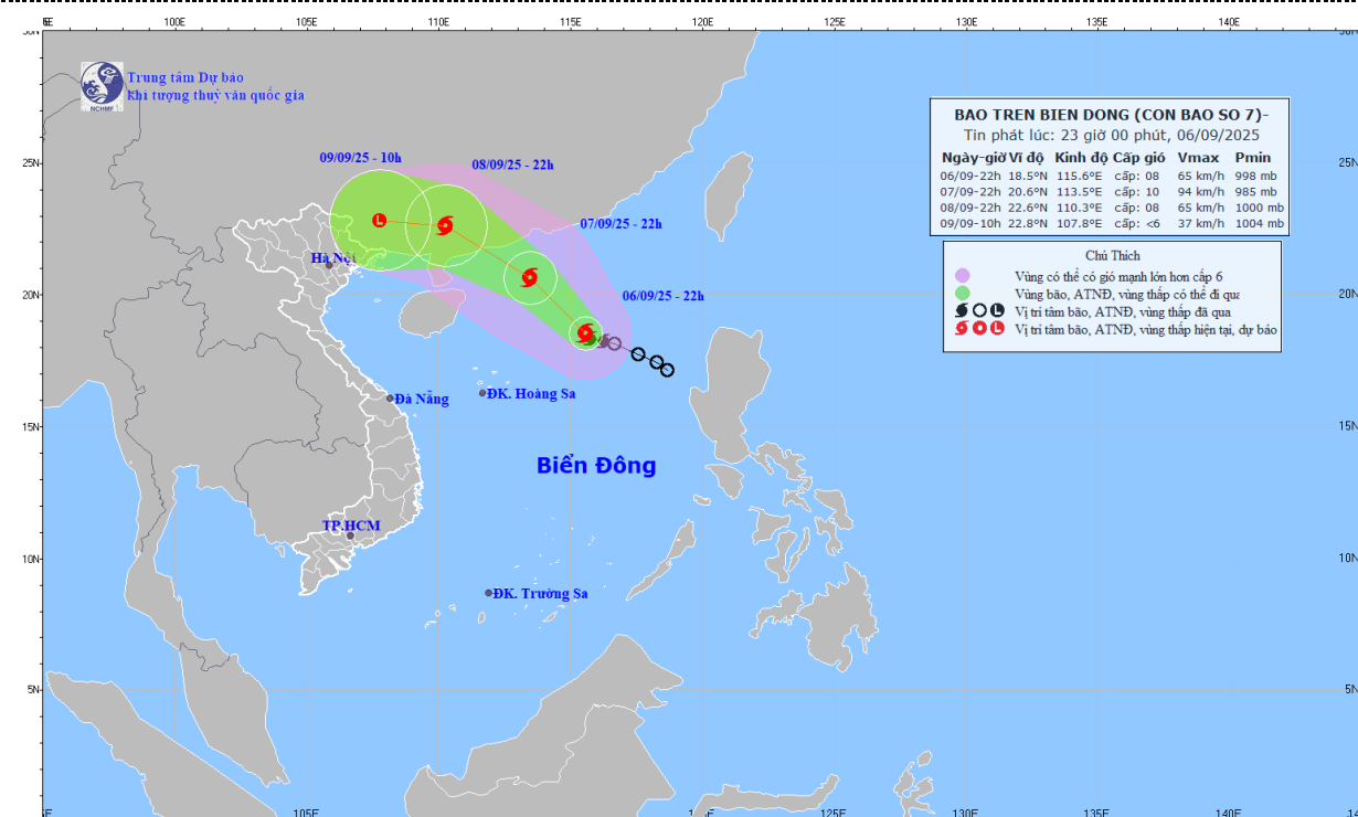
Hình1. Bản đồ dự báo quỹ đạo và cường độ bão lúc 23h00 ngày 06/9/2025
