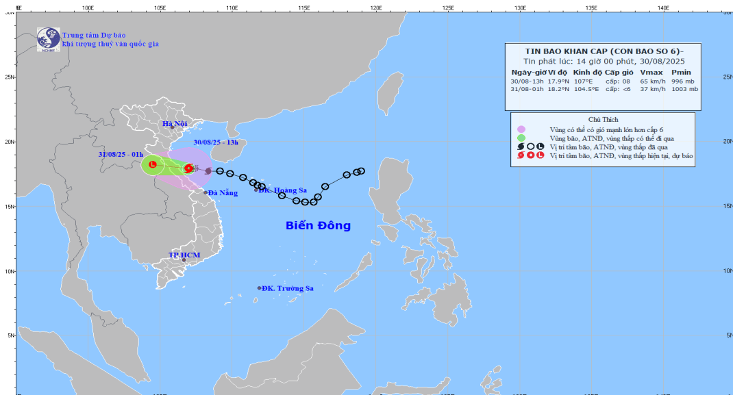
Hình1. Bản đồ dự báo quỹ đạo và cường độ Bão phát lúc 14h00 ngày 30/8/2025 (Nguồn: Trung tâm dự báo KTTV quốc gia)
