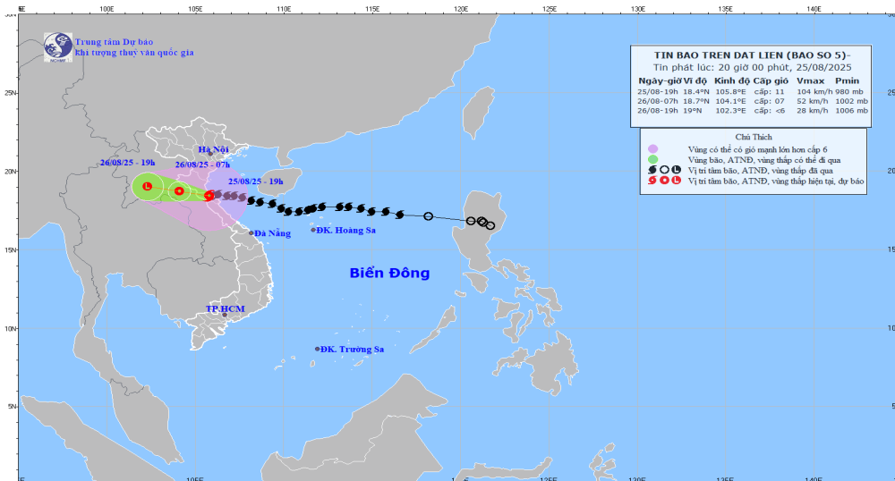
Hình1. Bản đồ dự báo quỹ đạo và cường độ bão số 05 phát lúc 20h00 ngày 25/8/2025 (Nguồn: Trung tâm dự báo KTTV quốc gia)
