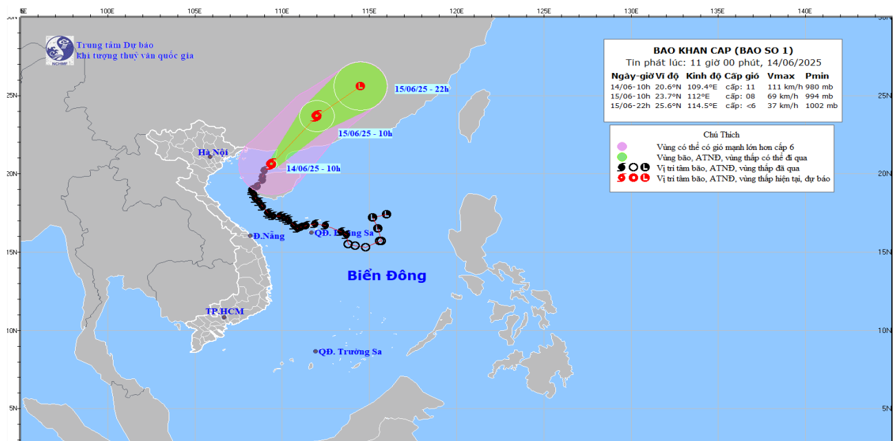
Hình1. Bản đồ dự báo quỹ đạo và cường độ bão số 01 lúc 11h00 ngày 14/6/2025
