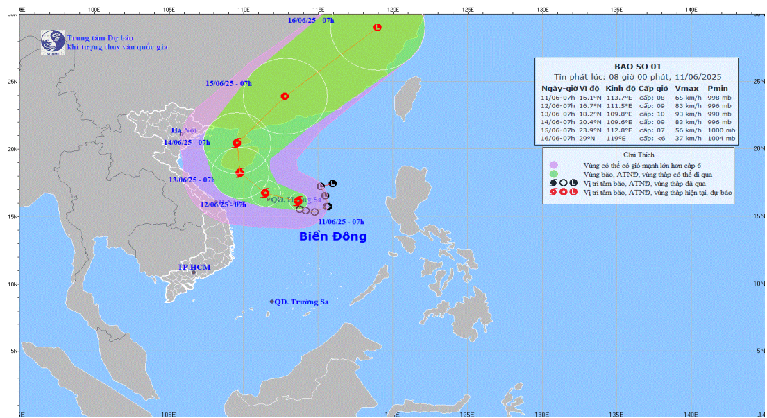
Hình1. Bản đồ dự báo quỹ đạo và cường độ bão số 01 lúc 08h00 ngày 11/6/2025
