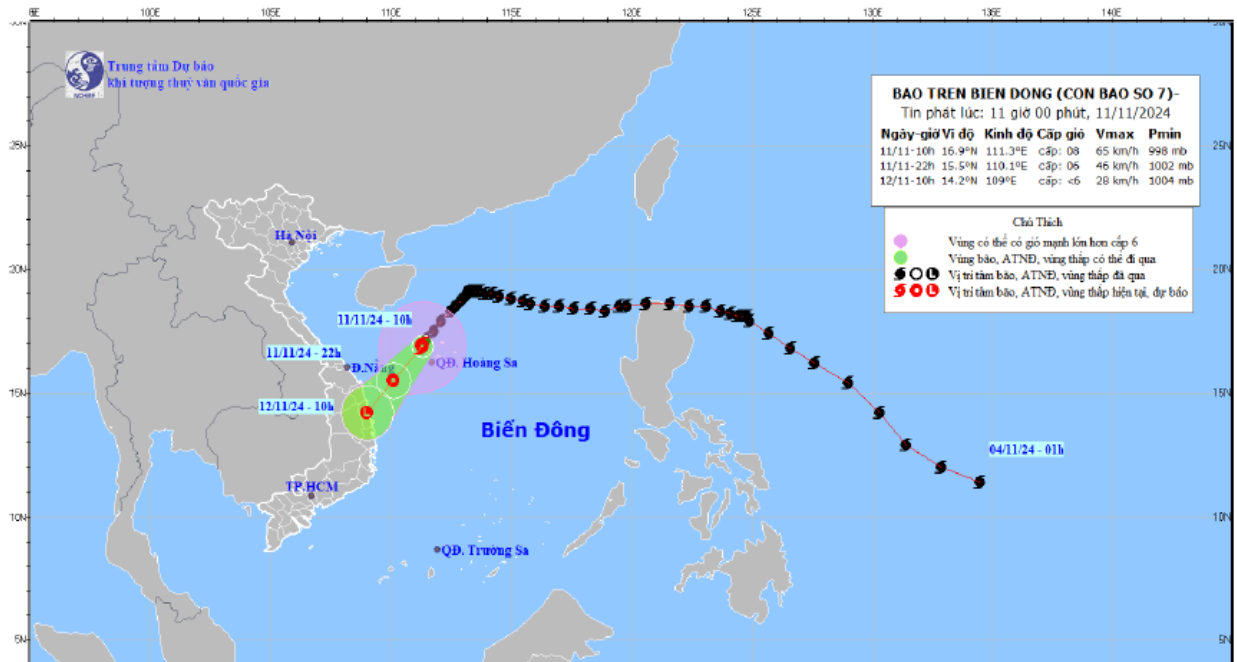
Bản đồ dự báo quỹ đạo và cường độ của bão số 07, phát lúc 11h00, ngày 11/11/2024
