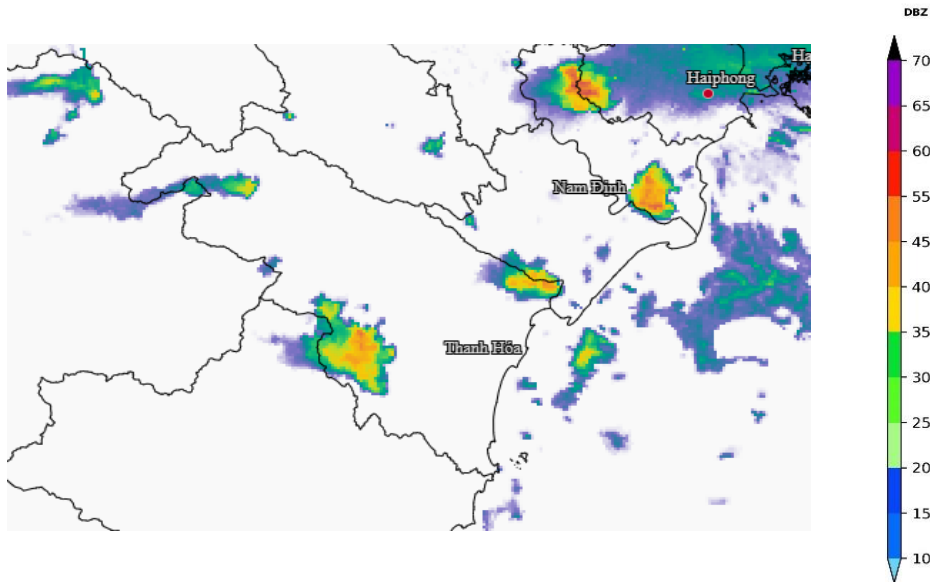
Hình 1: Ảnh radar thời tiết tỉnh Thanh Hoá
