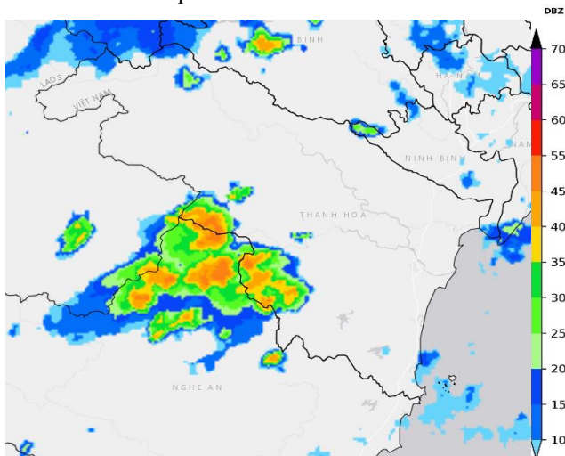
Sản phẩm của Radar lúc 14h10
