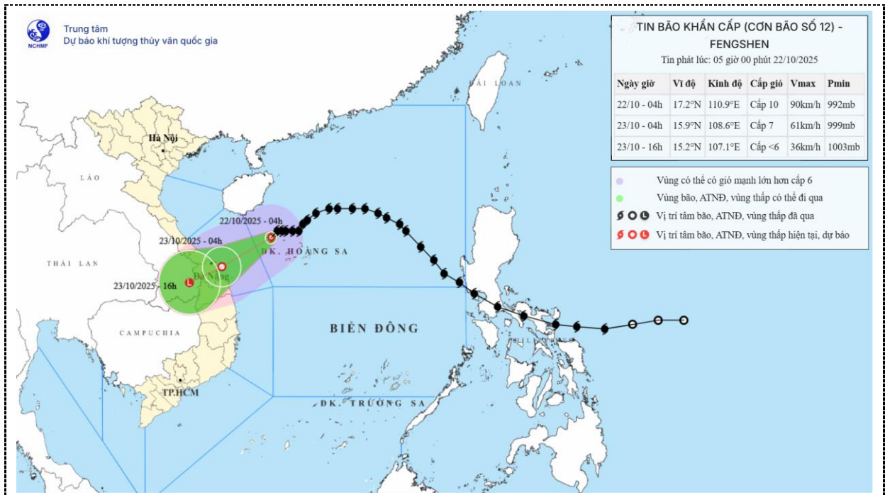
Hình 1. Bản đồ dự báo quỹ đạo và cường độ bão phát lúc 05h00 ngày 22/10/2025
