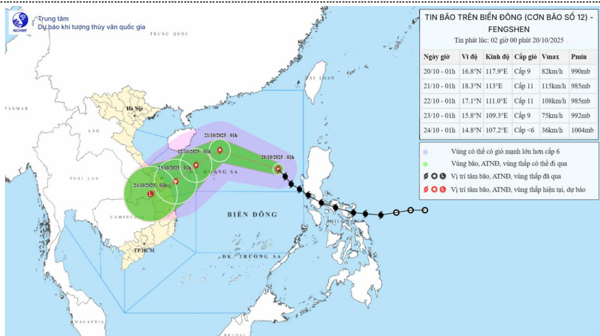
Hình 1. Bản đồ dự báo quỹ đạo và cường độ bão số 12 phát lúc 02h00 ngày 20/10/2025
