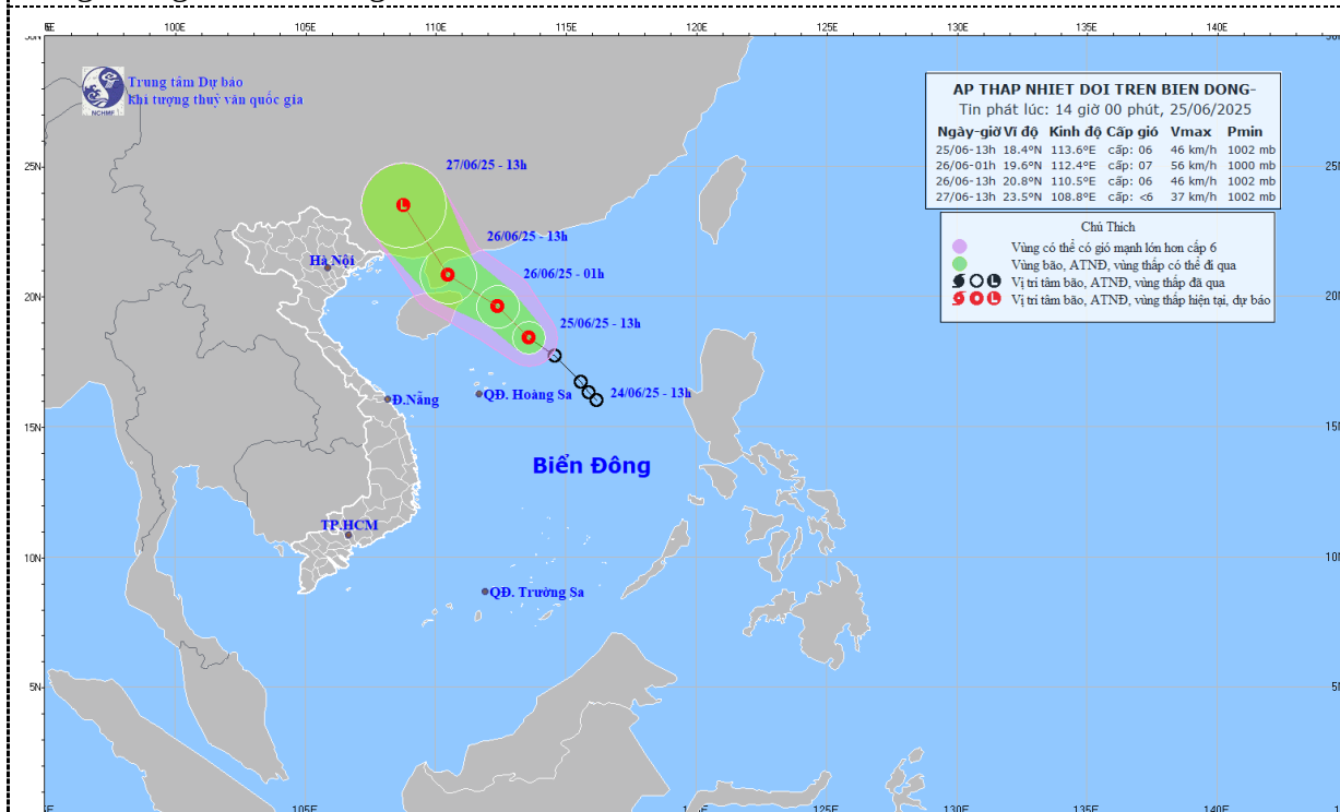
Hình1. Bản đồ dự báo quỹ đạo và cường độ áp thấp nhiệt đới lúc 14h00 ngày 25/6/2025
