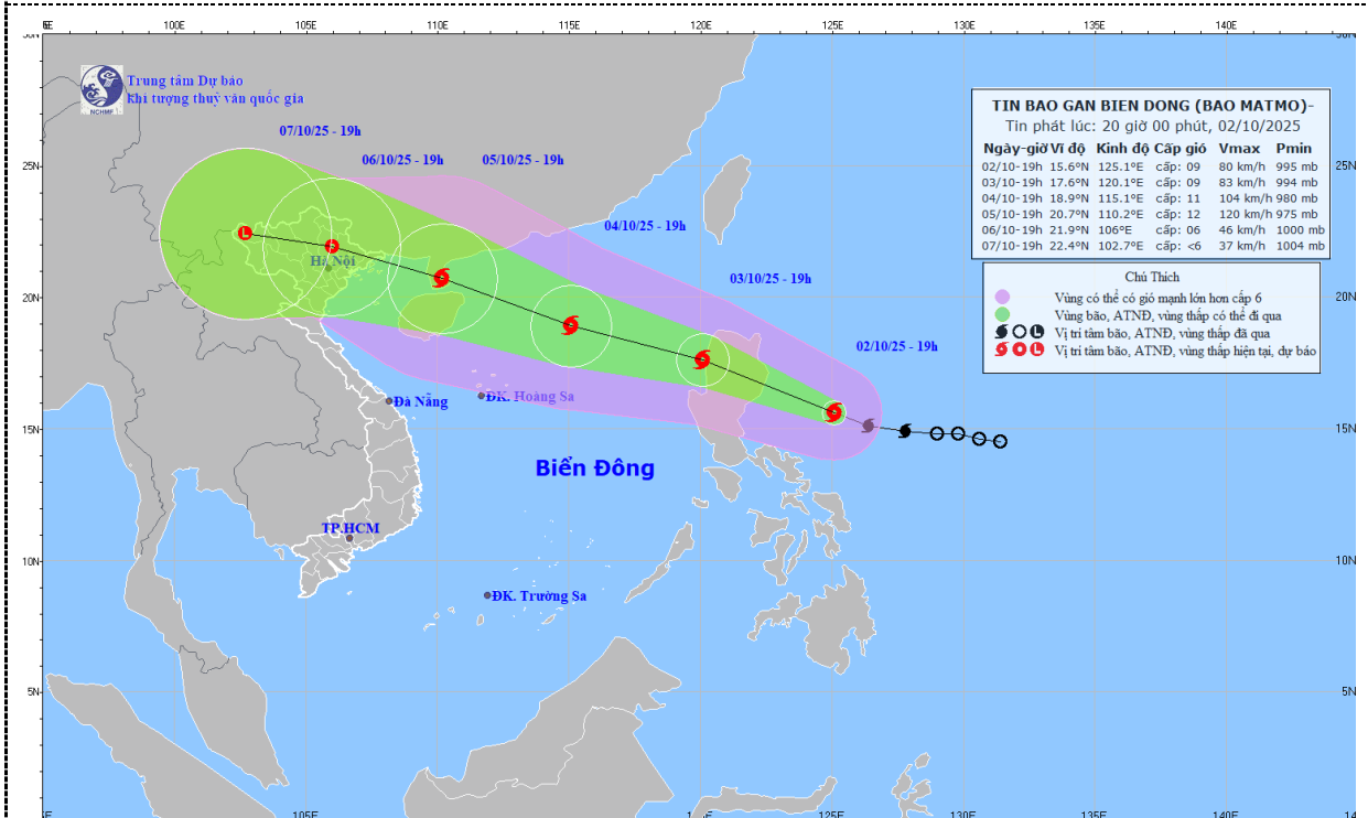
Hình1. Bản đồ dự báo quỹ đạo và cường độ bão phát lúc 20h00 ngày 02/10/2025
