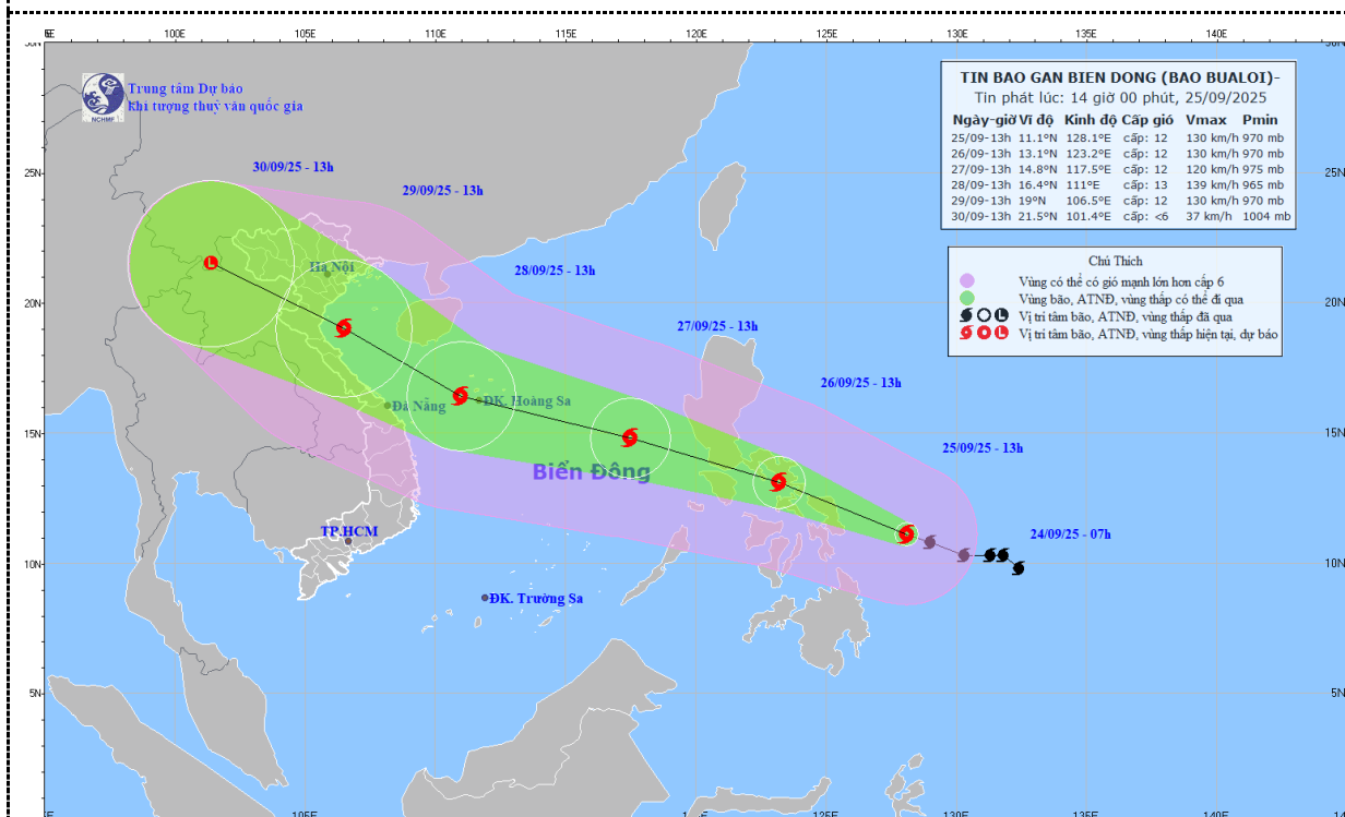
Hình1. Bản đồ dự báo quỹ đạo và cường độ bão BUALOI phát lúc 14h00 ngày 25/9/2025
