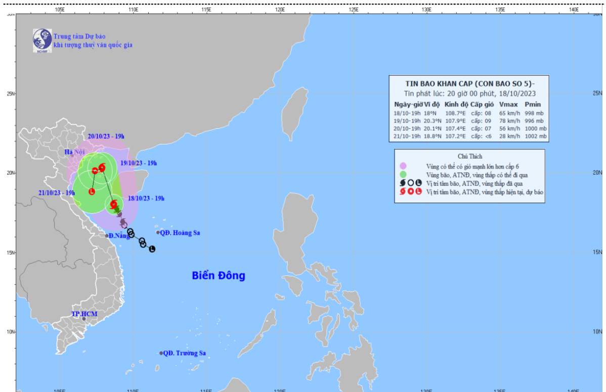
Bản đồ dự báo quỹ đạo và cường độ bão, phát lúc 20h00 ngày 18/10/2023
