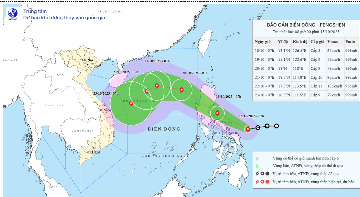
Hình 1. Bản đồ dự báo quỹ đạo và cường độ bão FENGSHEN phát lúc 08h00 ngày 18/10/2025
