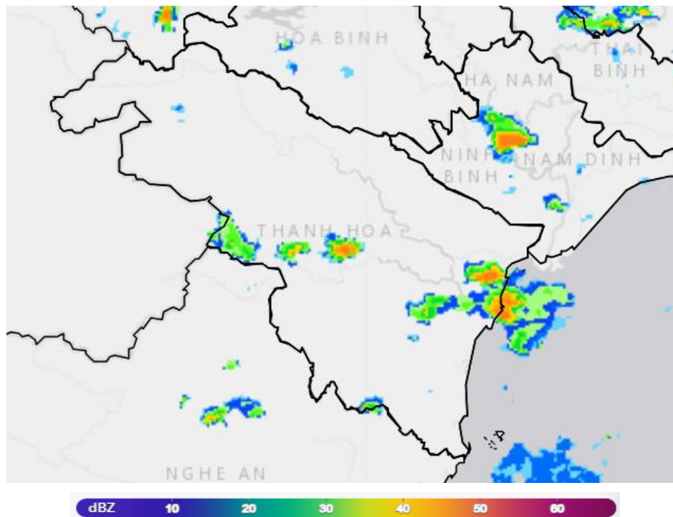
Hình 1: Ảnh radar thời tiết tỉnh Thanh Hoá
