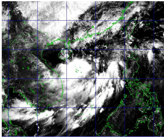
Hình ảnh mây vệ tinh, lúc 10h00 ngày 30/05/2024
