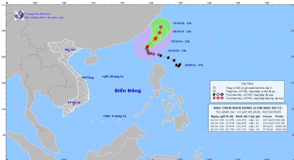
Bản đồ dự báo quỹ đạo và cường độ của bão, phát lúc 14h00, ngày 02/10/2024
