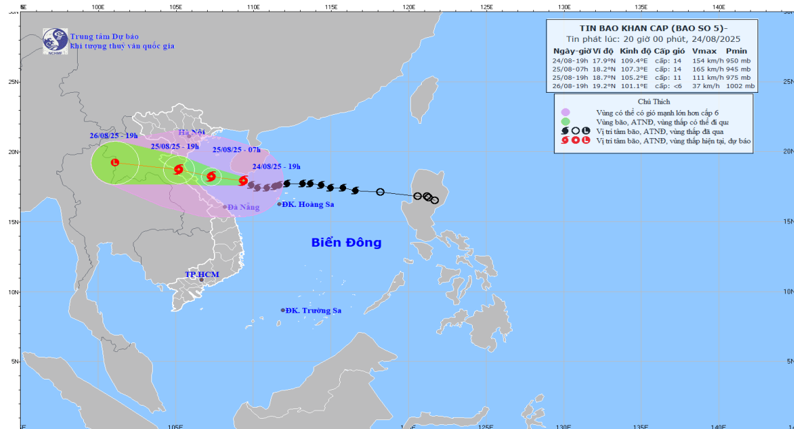
Hình1. Bản đồ dự báo quỹ đạo và cường độ bão số 05 phát lúc 20h00 ngày 24/8/2025
