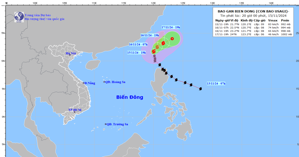
Bản đồ dự báo quỹ đạo và cường độ của bão USAGI, phát lúc 20h00, ngày 15/11/2024
