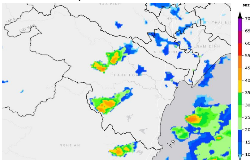
Sản phẩm của Radar lúc 14h10
