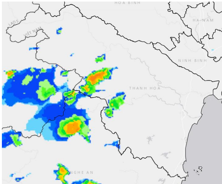
Sản phẩm của Radar lúc 14h20
