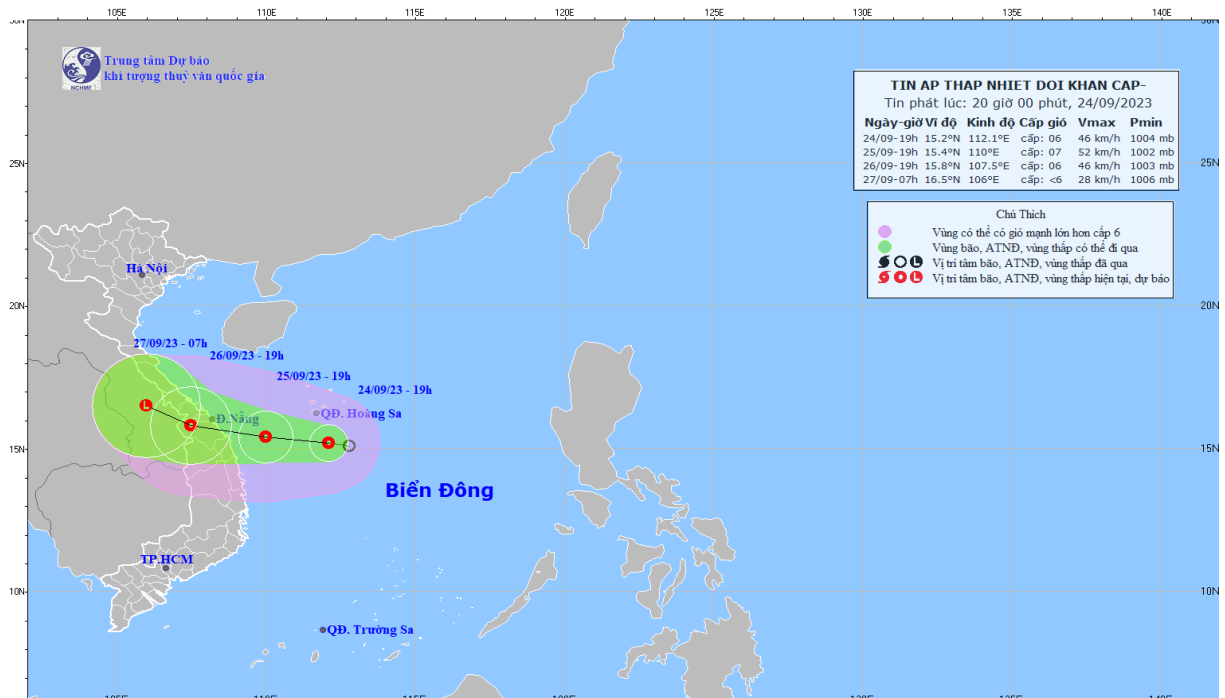
Bản đồ dự báo quỹ đạo và cường độ ATND trên Biển Đông, phát lúc 20h00 ngày 24/9/2023
